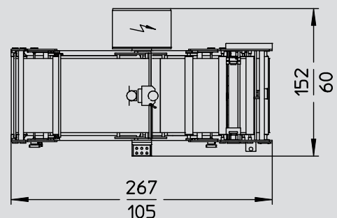
Grundaufbau PFS
