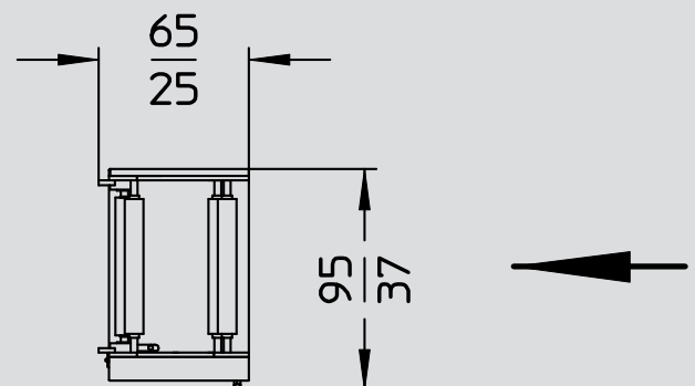
Grundaufbau CM80
