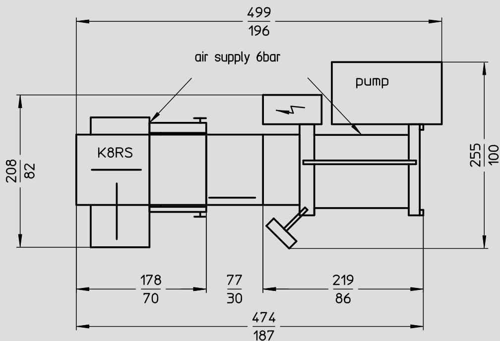
Plan d'implantation K8RS avec margeur à palette
